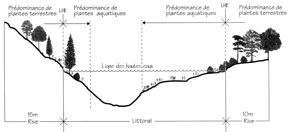
Figure 17 Ligne des hautes eaux (LHE)
