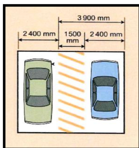
Figure 5 Aménagement d'un espace de stationnement
