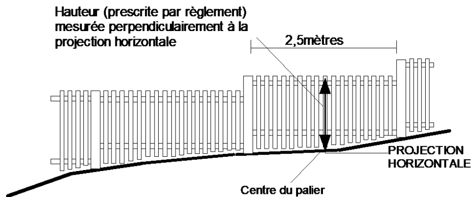
Figure 3 Hauteur autorisée pour une clôture privée selon sa localisation
