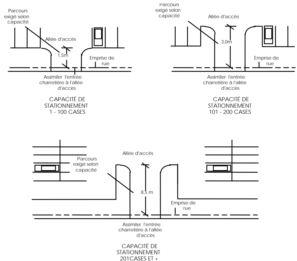
Figure 1 Aménagement d'une allée d'accès
